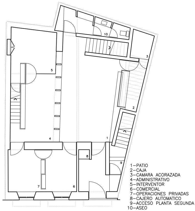
PLANTA BAJA
