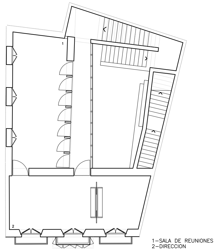
PLANTA PRIMERA
