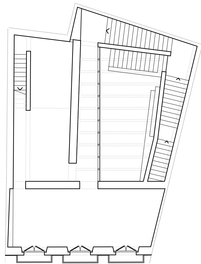
PLANTA SEGUNDA
