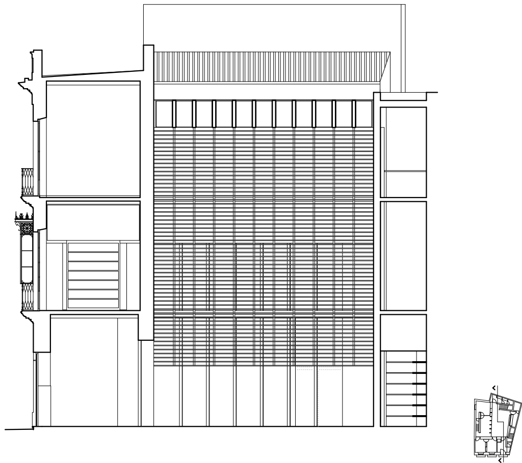
SECCION LONGITUDINAL 2
