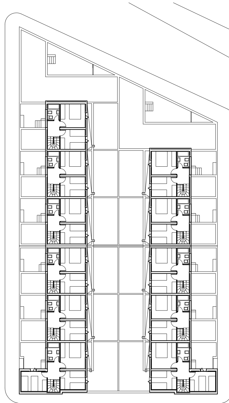
PLANTA PRIMERA
