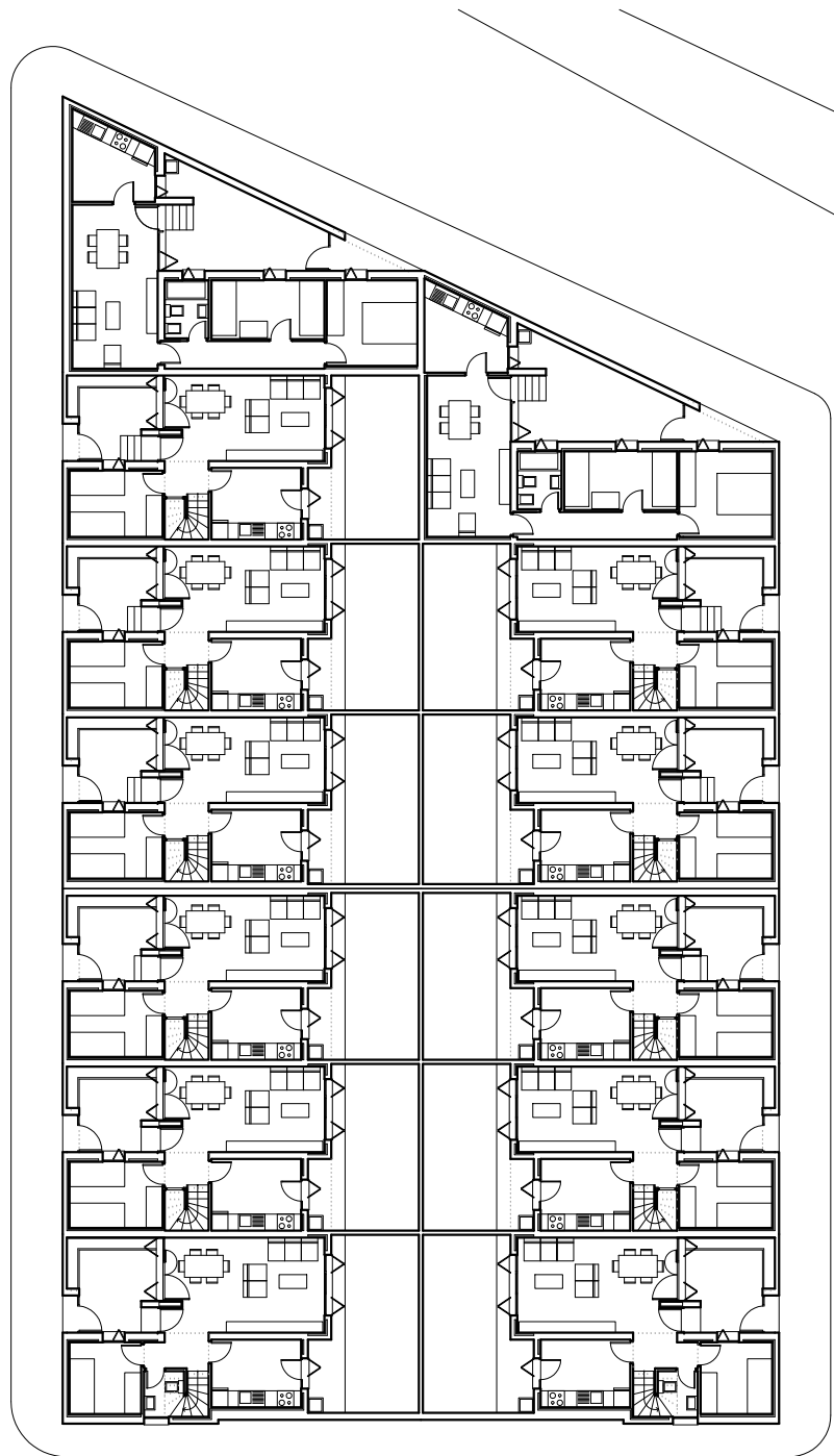
PLANTA BAJA
