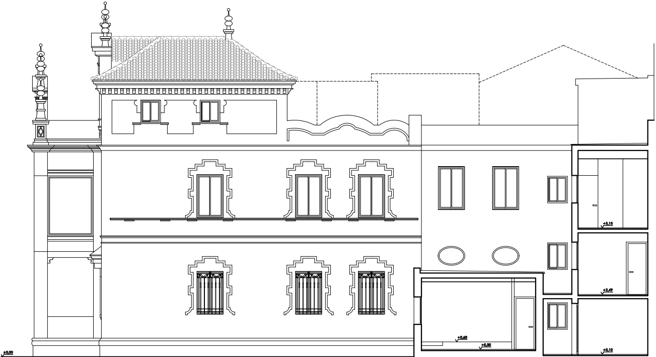
ALZADO ESTE Cotas en metros.
