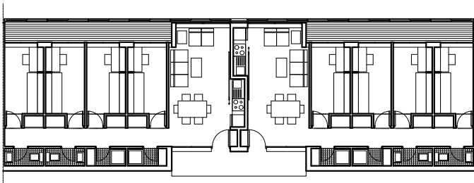
TIPO 4 DORMITORIOS
