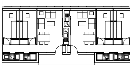
TIPO 2 DORMITORIOS
