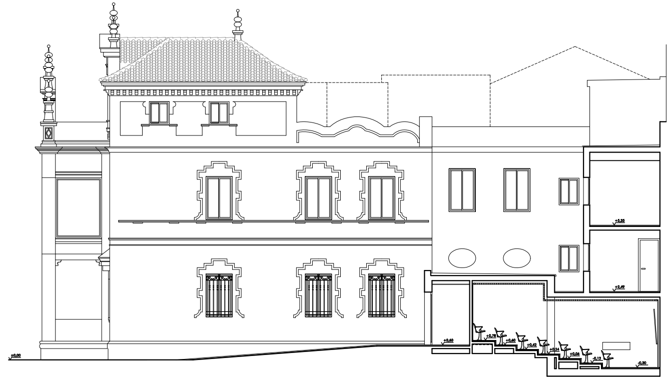
ALZADO ESTE Cotas en metros
