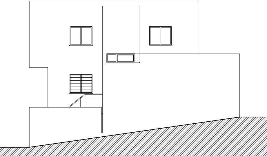
ALZADO 3 - ALZADO LATERAL SUROESTE
