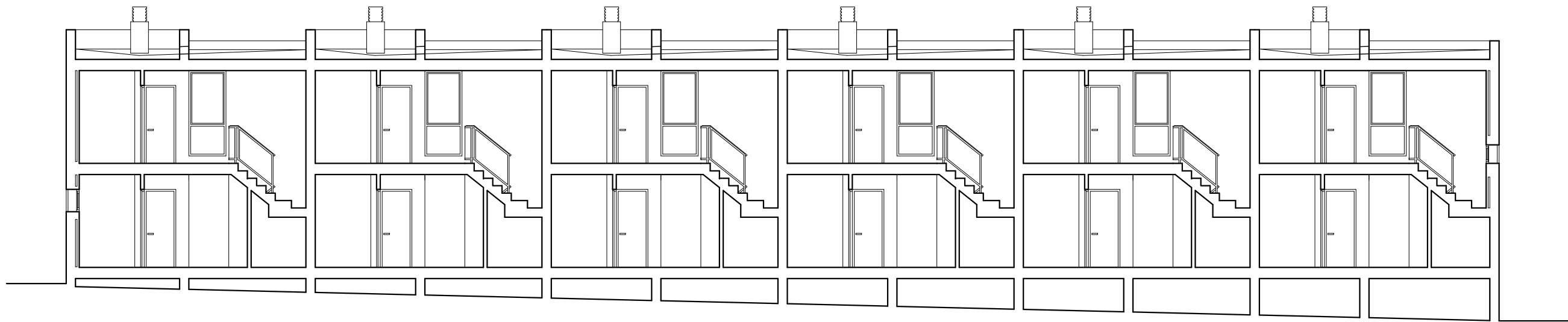
SECCION LONGITUDINAL A-A
