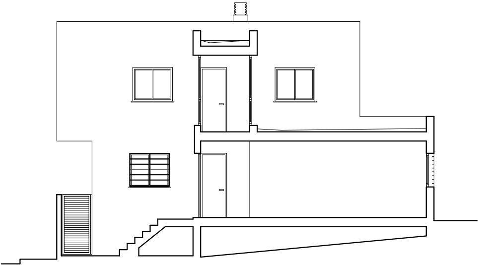
SECCION TRASVERSAL C-C
