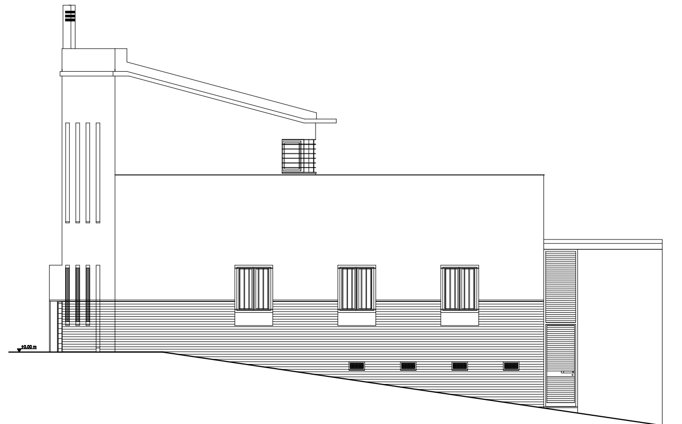
ALZADO EXTERIOR B-B
