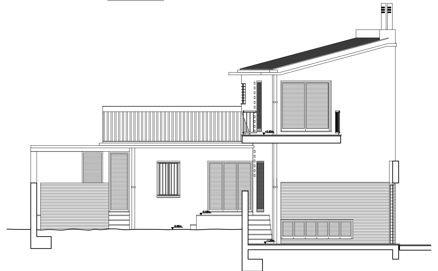
ALZADO INTERIOR D-D
