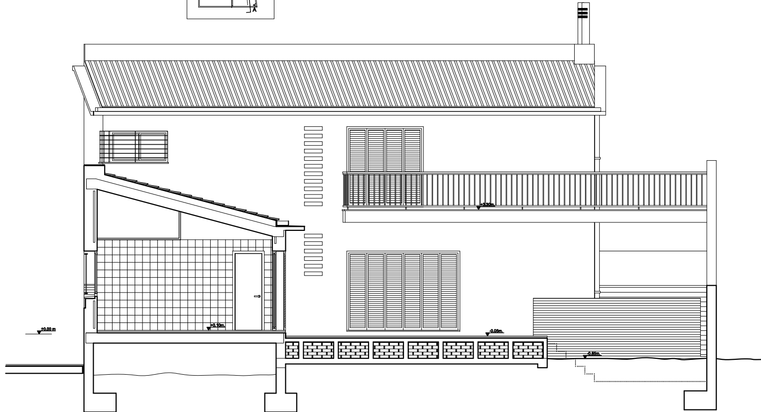
SECCION C-C
