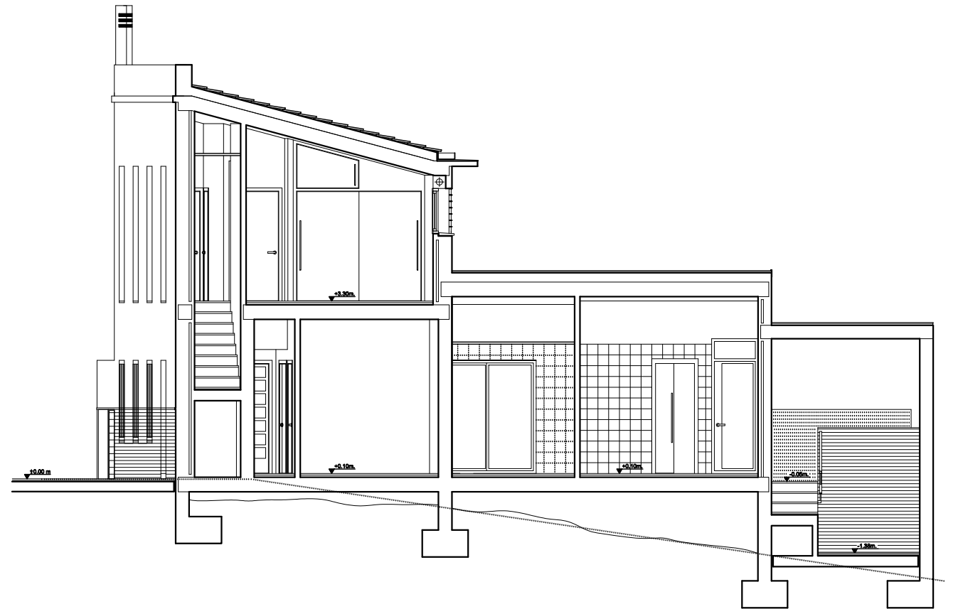
SECCION B-B
