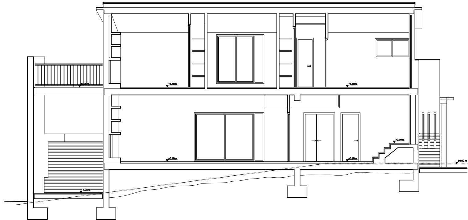
SECCION A-A
